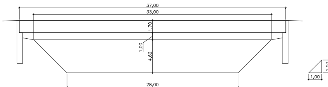
Figura 8 - Seção Determinada e cota para instalação da Ponte
