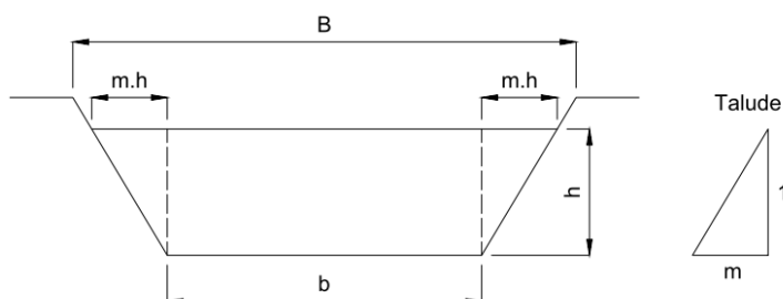
Figura 7 - Geometria da seção a ser calculada
